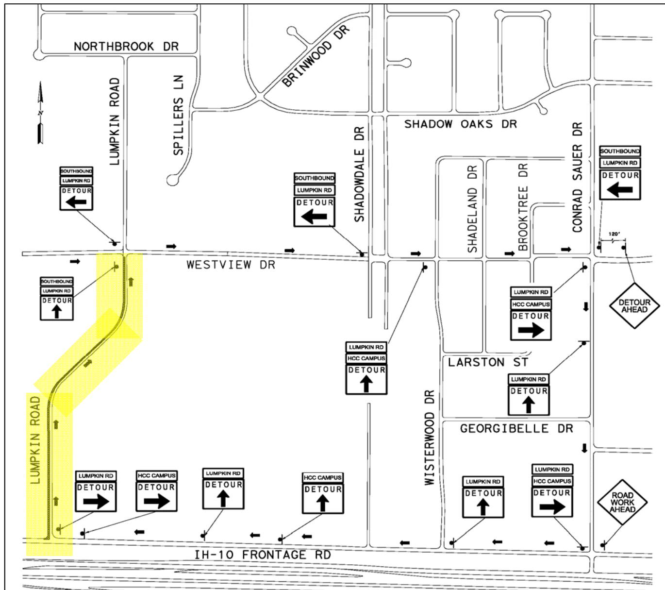
PHASE 1 DETOUR PLAN
