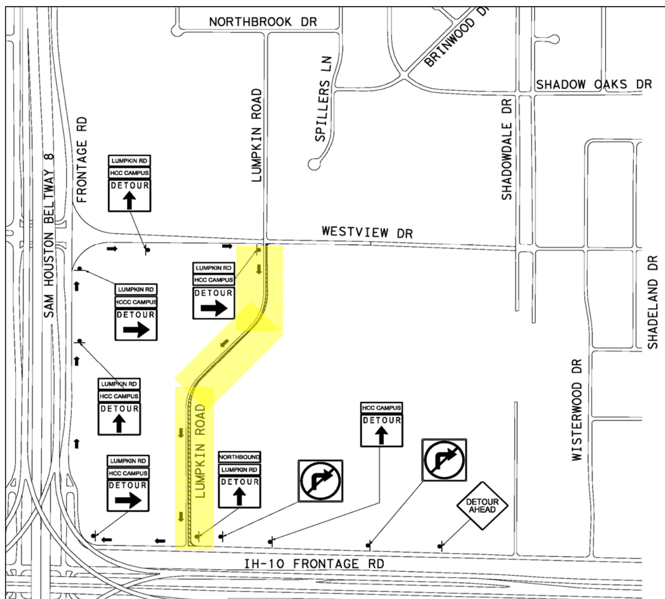
PHASE 2 DETOUR PLAN
